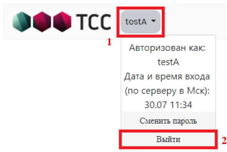
Рисунок 7 – Кнопка «Выйти»
